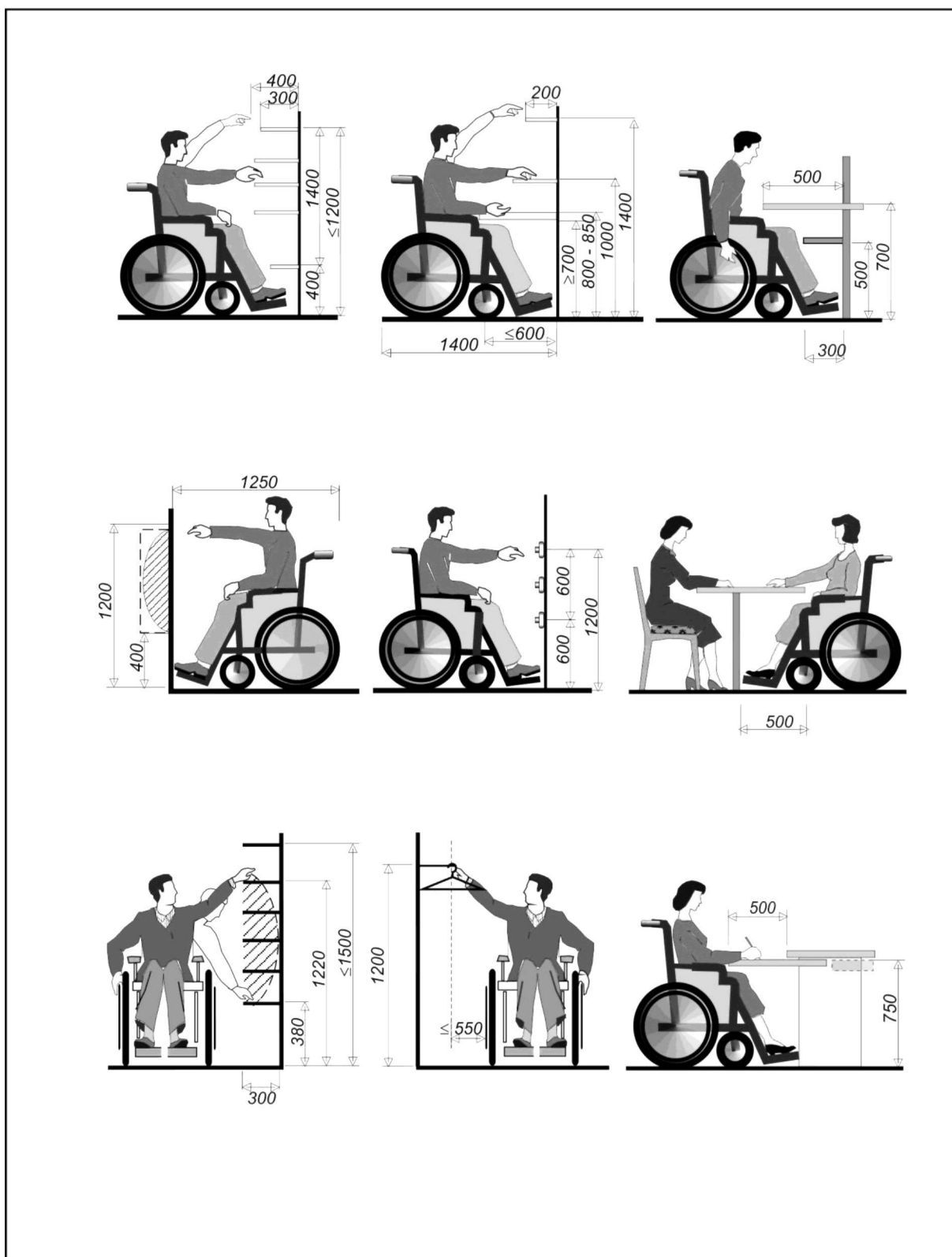
Рисунок Г.3 Параметры досягаемости в месте получения услуги
