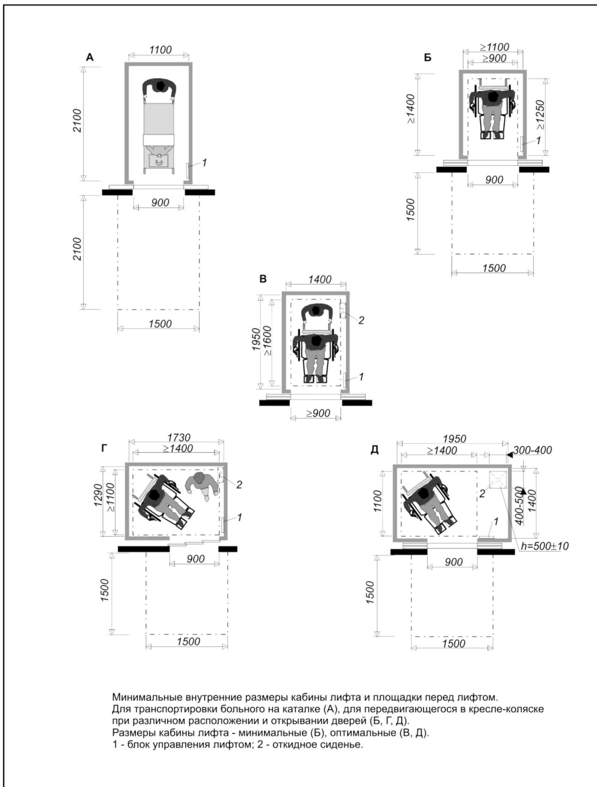
Рисунок В.23 Габариты лифтов
