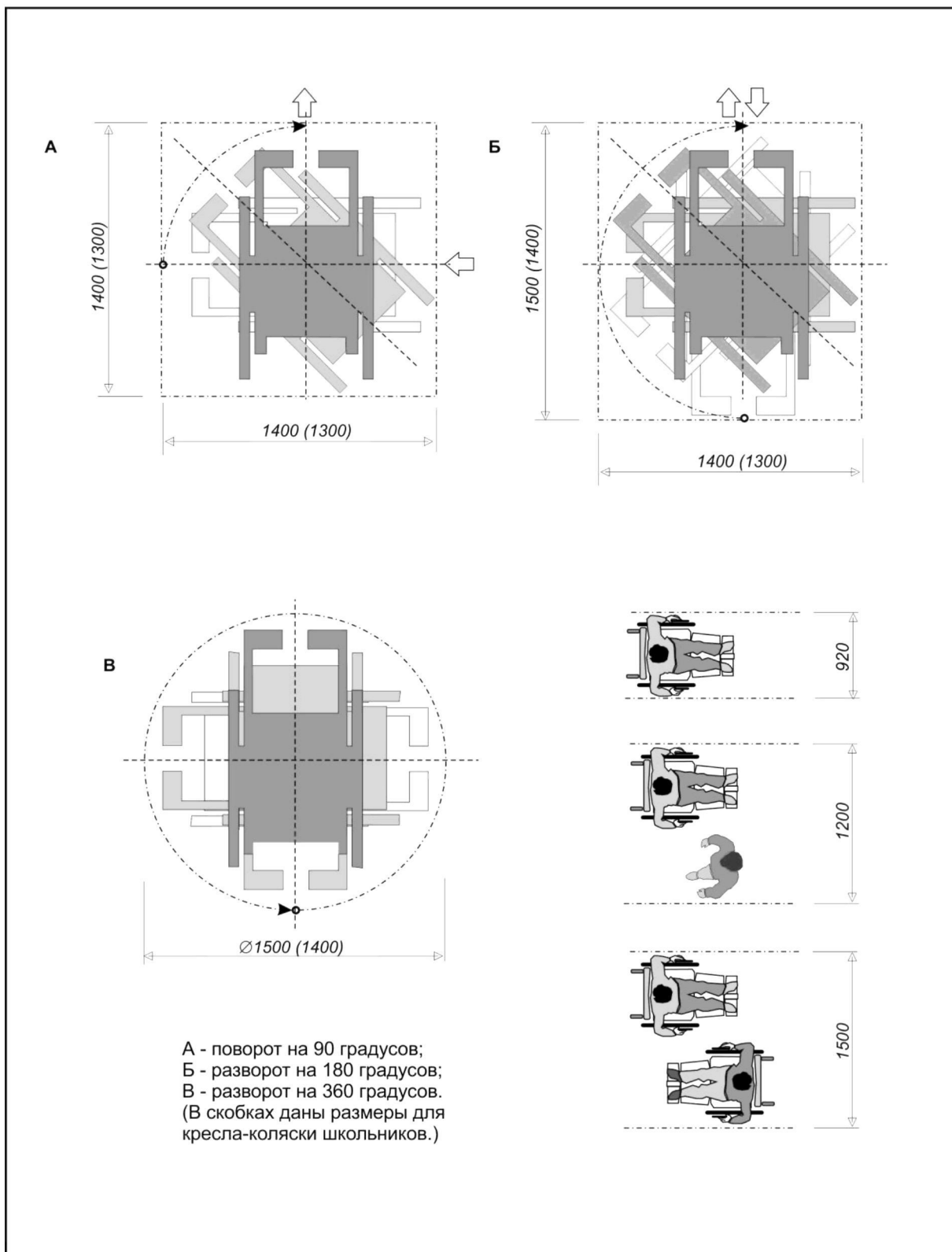
Рисунок В.3 Параметры занимаемой зоны при вращении и движении МГН на кресле-коляске
