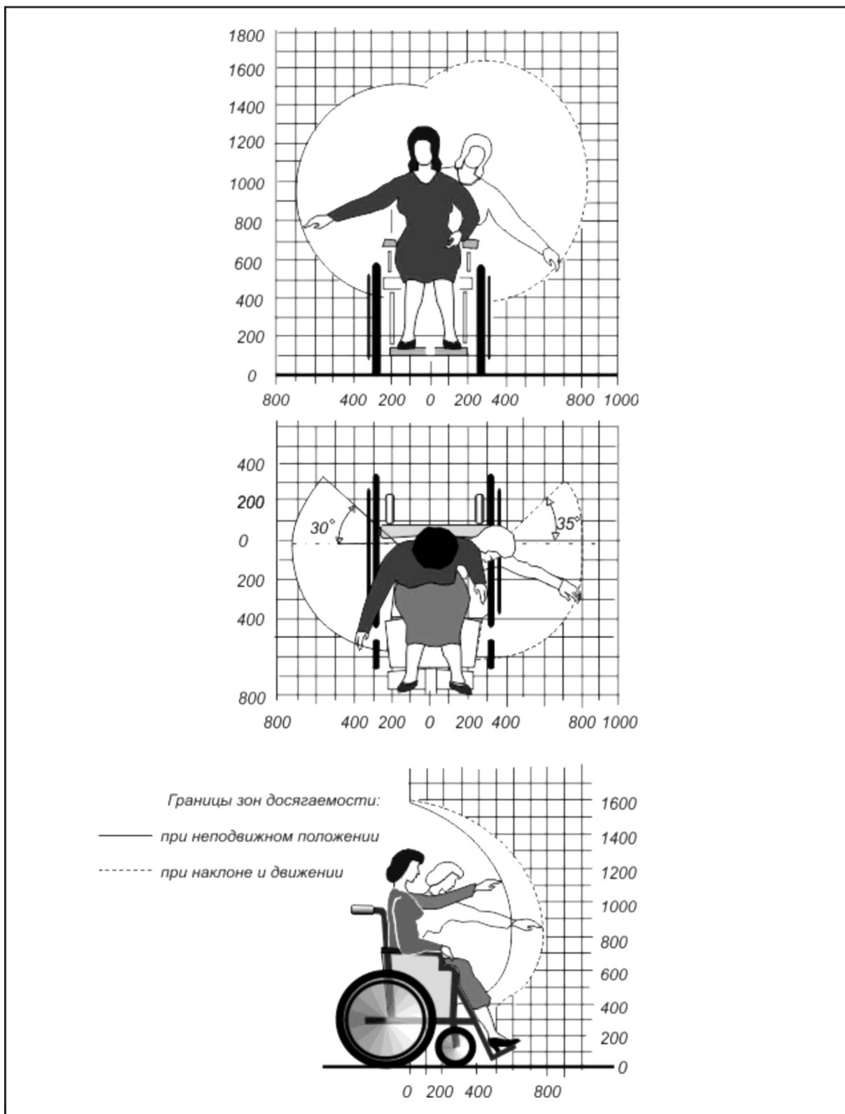
Рисунок Г.2 Зоны досягаемости инвалидов на кресле-коляске для женщин
