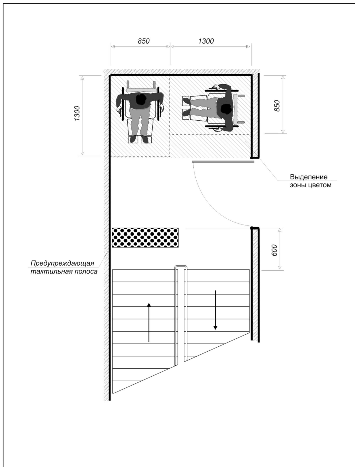
Рисунок В.20 Зона-накопитель для инвалидов на лестничной клетке при эвакуации
