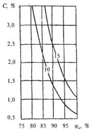
Рисунок Ш.2 - Изолинии сорбционного влагосодержания керамзитобетона \rho_0 = 1200 \text{ кг/м}^3 , содержащего хлорид калия, при
