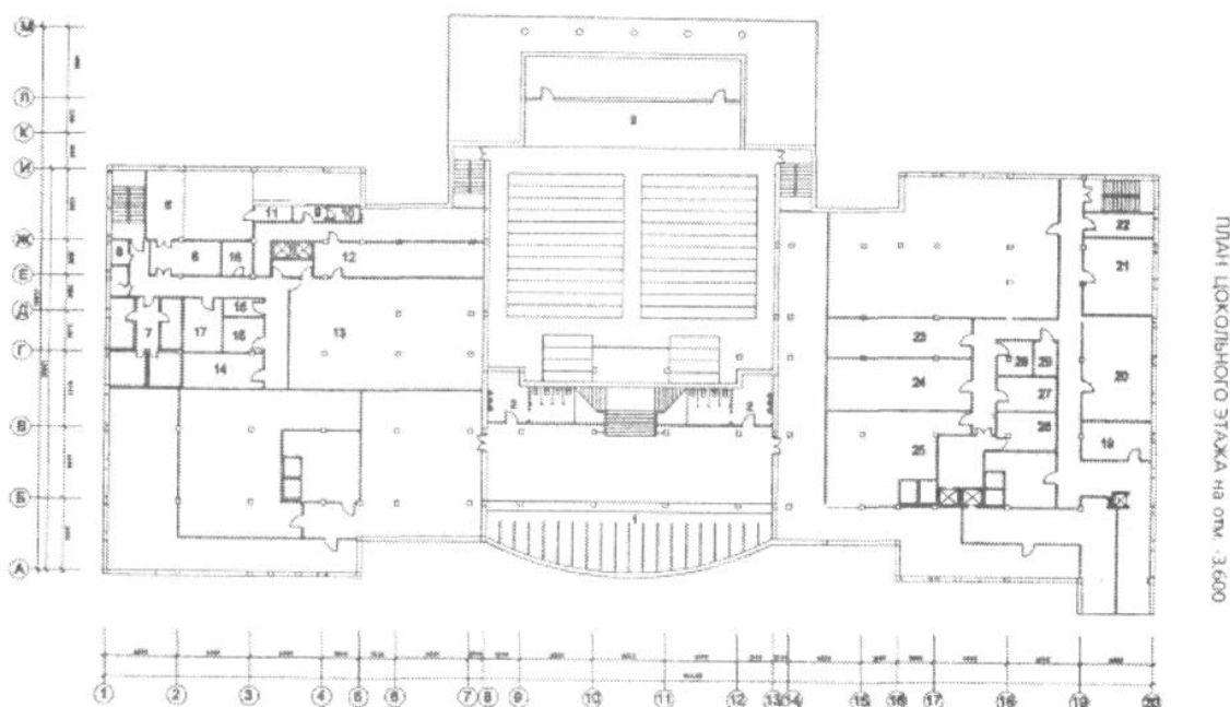
Рисунок Я.2 - План цокольного этажа
