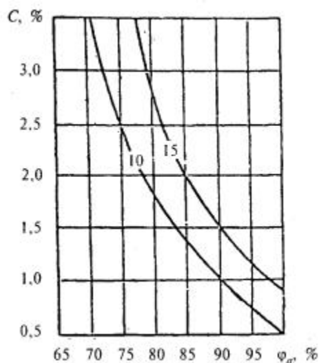
Рисунок Ш.1 - Изолинии сорбционного влагосодержания керамзитобетона \rho_0 = 1200 \text{ кг/м}^3 , содержащего хлорид натрия, при изменении относительной влажности воздуха \varphi_a , %, и массового солесодержания C , %
