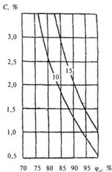
Рисунок Ш.6 - Изолинии сорбционного влагосодержания керамзитобетона \rho_0 = 1200 \text{ кг/м}^3 , содержащего NaCl - 30 %, KCl - 60 %, \text{MgCl}_2 - 10 %, при изменении относительной влажности
