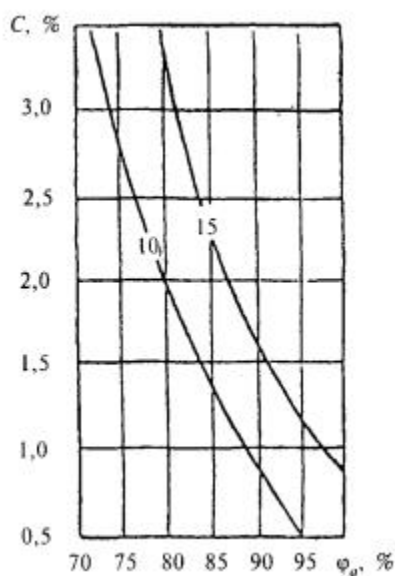
Рисунок Ш.4 - Изолинии сорбционного влагосодержания керамзитобетона \rho_0 = 1200 \text{ кг/м}^3 , содержащего NaCl - 60 %, KCl - 30 %, \text{MgCl}_2 - 10 %, при изменении относительной влажности
