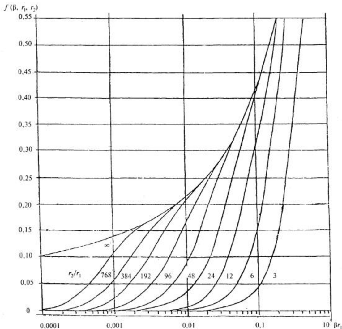
Рисунок П.1 - Функция f(b, r_1, r_2)
