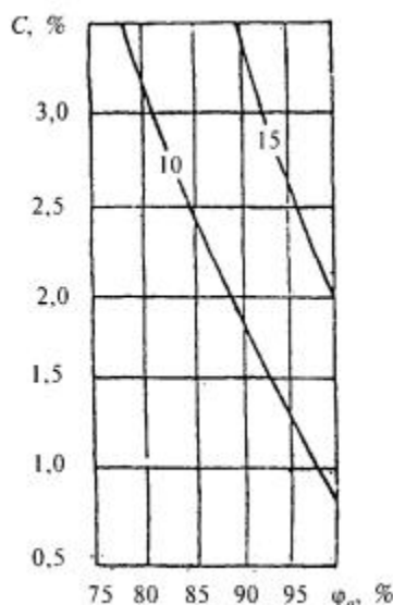
Рисунок Ш.3 - Изолинии сорбционного влагосодержания керамзитобетона \rho_0 = 1200 \text{ кг/м}^3 , содержащего хлорид магния, при изменении относительной влажности воздуха j_a , %, и массового солесодержания C , %
