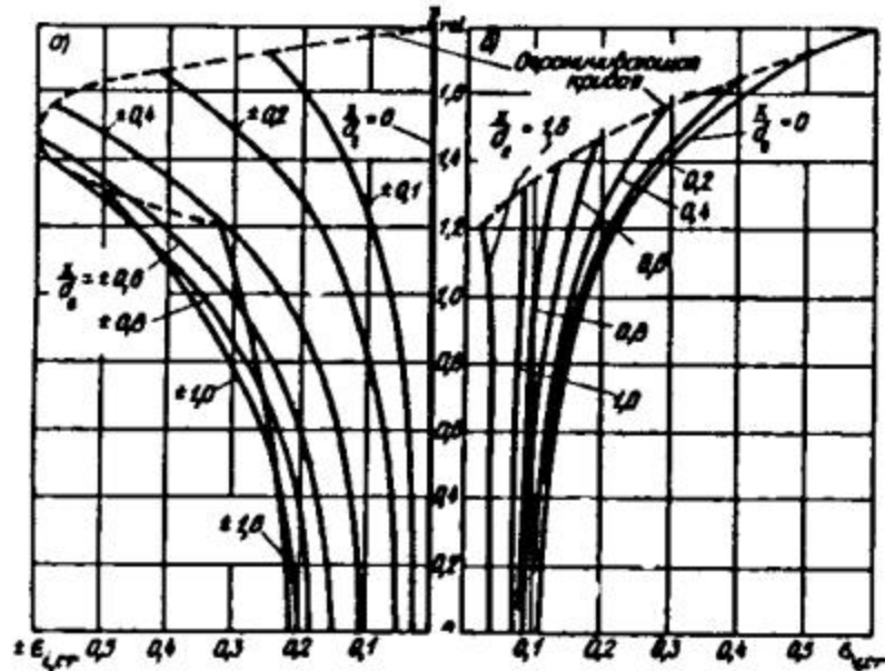
Рис. 25. Графики значений инерционного e_{i,cr} и скоростного e_{v,cr} коэффициентов
