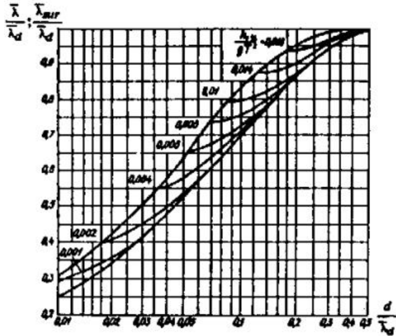
Рис. 4. Графики для определения значений
