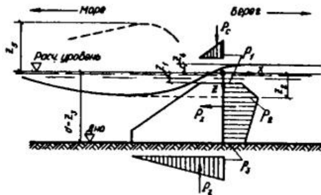
Рис. 26. Эпюры волнового давления на подводный волнолом
