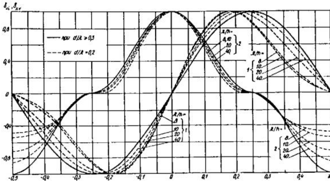
Рис. 18. Графики значений коэффициентов сочетания инерционного d_{xi} (графики 1) и скоростного d_{xv} (графики 2) компонентов горизонтальной линейной нагрузки от волн
