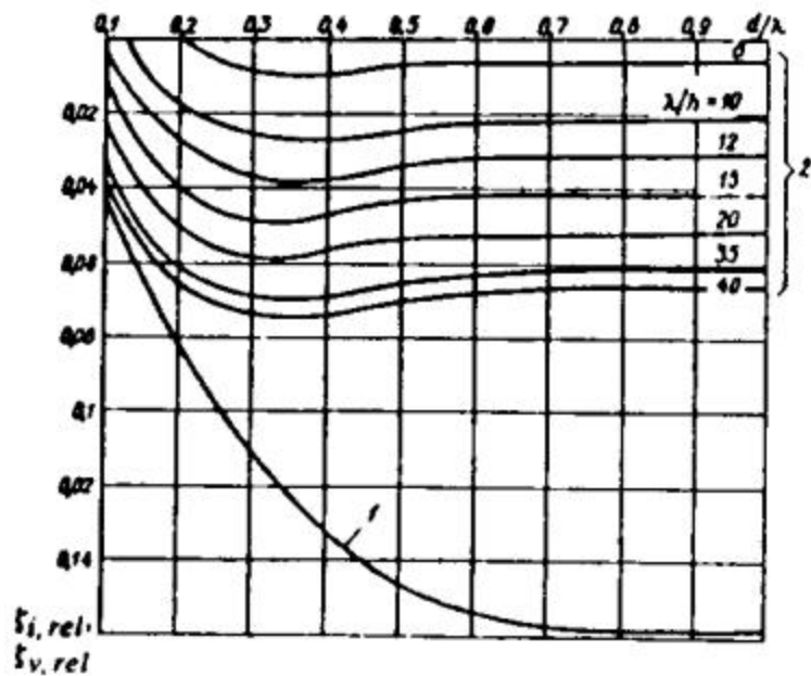
Рис. 21. Графики значений относительных координат
