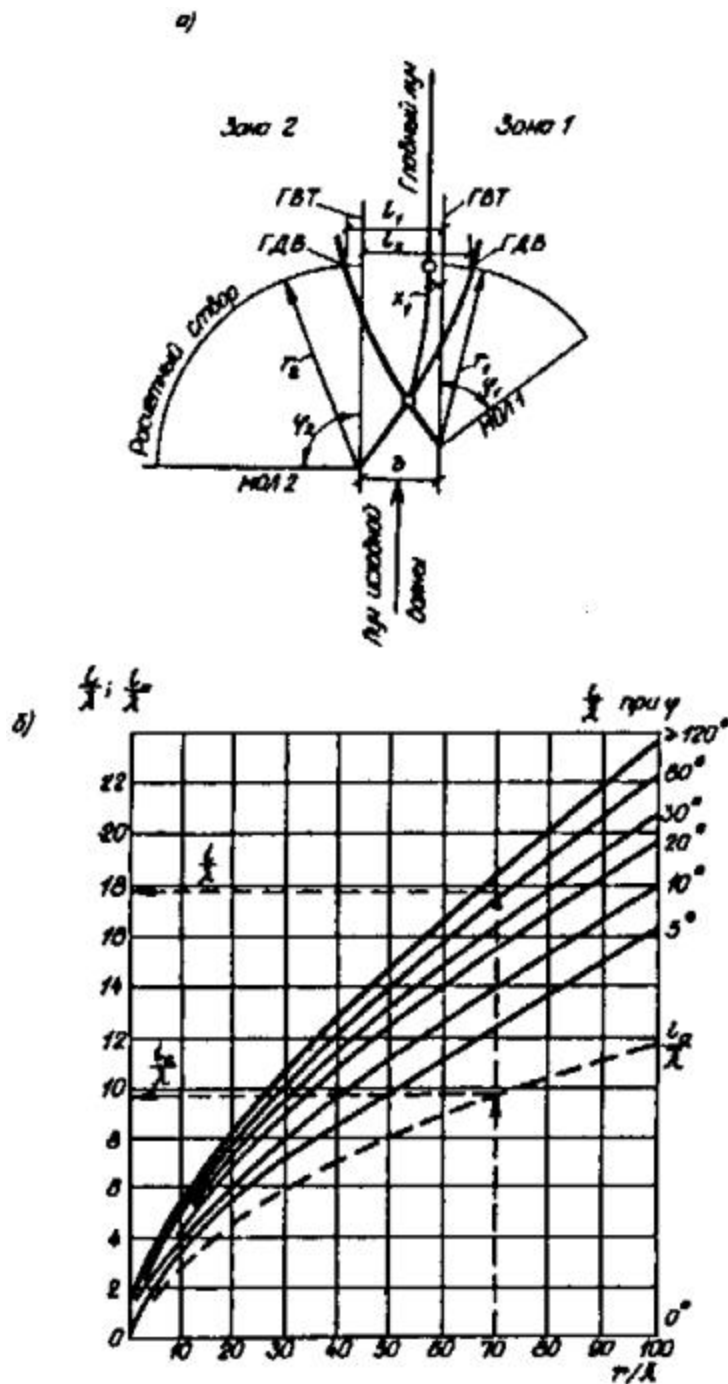
Рис. 9. Схема (а) и графики (б) для определения величин i и l_a
