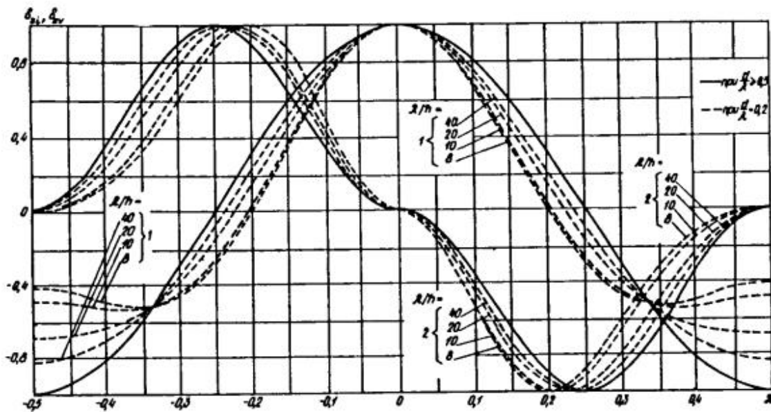
Рис. 23. Графики значений коэффициентов сочетания d_{zi} инерционного (графики 1) и d_{zv} - скоростного (графики 2) компонентов вертикальной линейной нагрузки от ВОЛН
