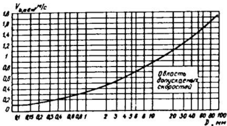
Рис. 7. График допускаемых значений неразмывающих донных скоростей
