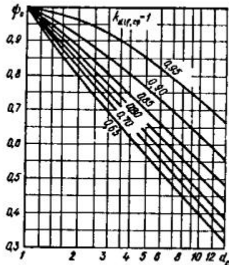
Рис. 8. Графики значений коэффициента u_c
