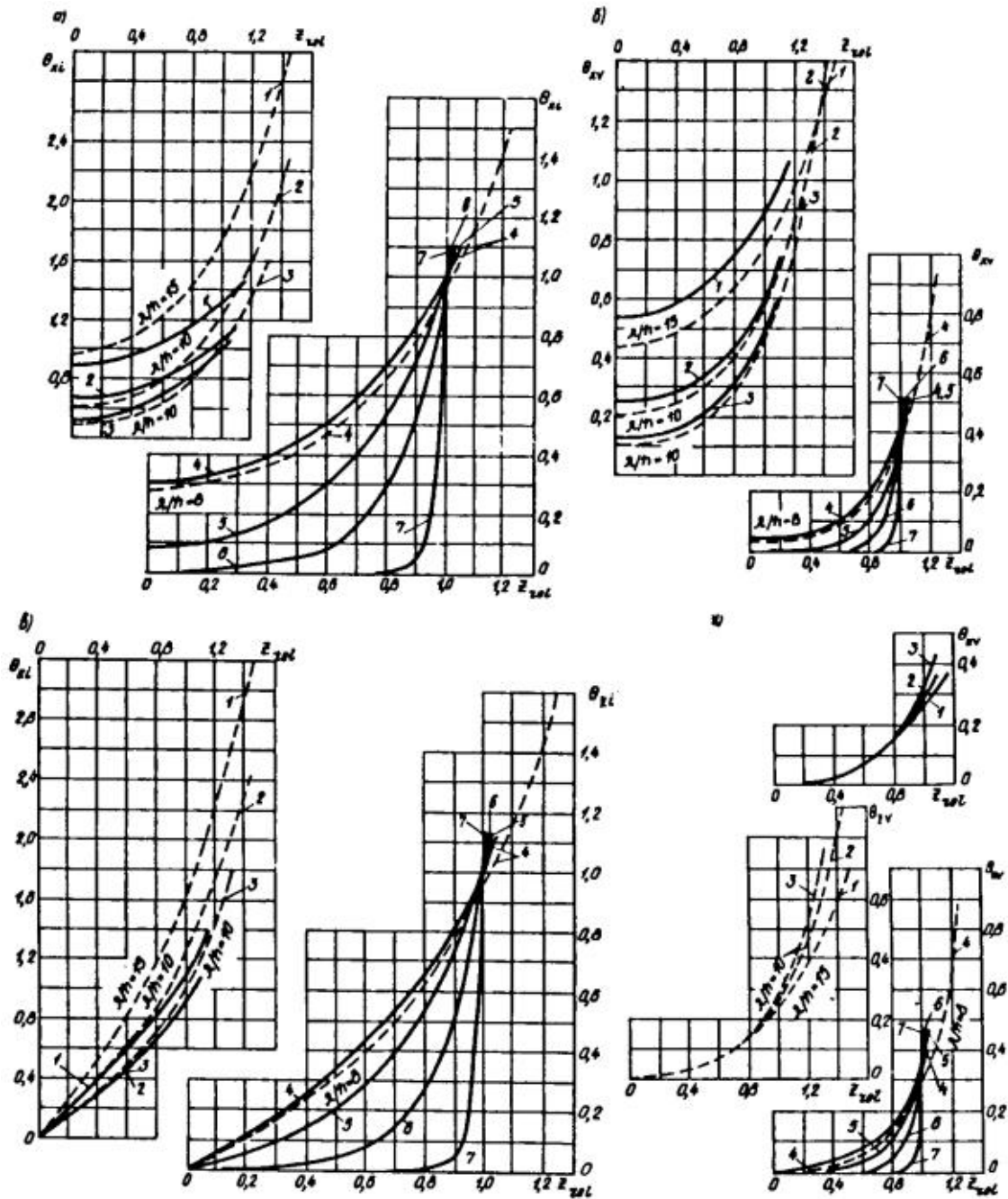
Рис. 19. Графики коэффициентов линейной нагрузки от волн q_{xi} , q_{xv} , q_{zv} при d/l :
