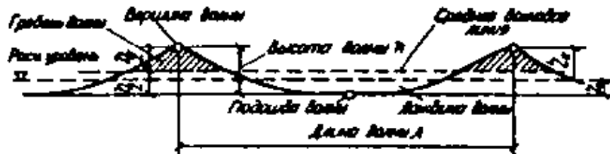
Профиль и элементы волны
