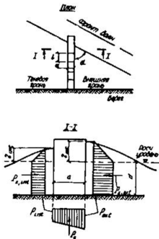
Рис. 30. Эпюры волнового давления на буну
