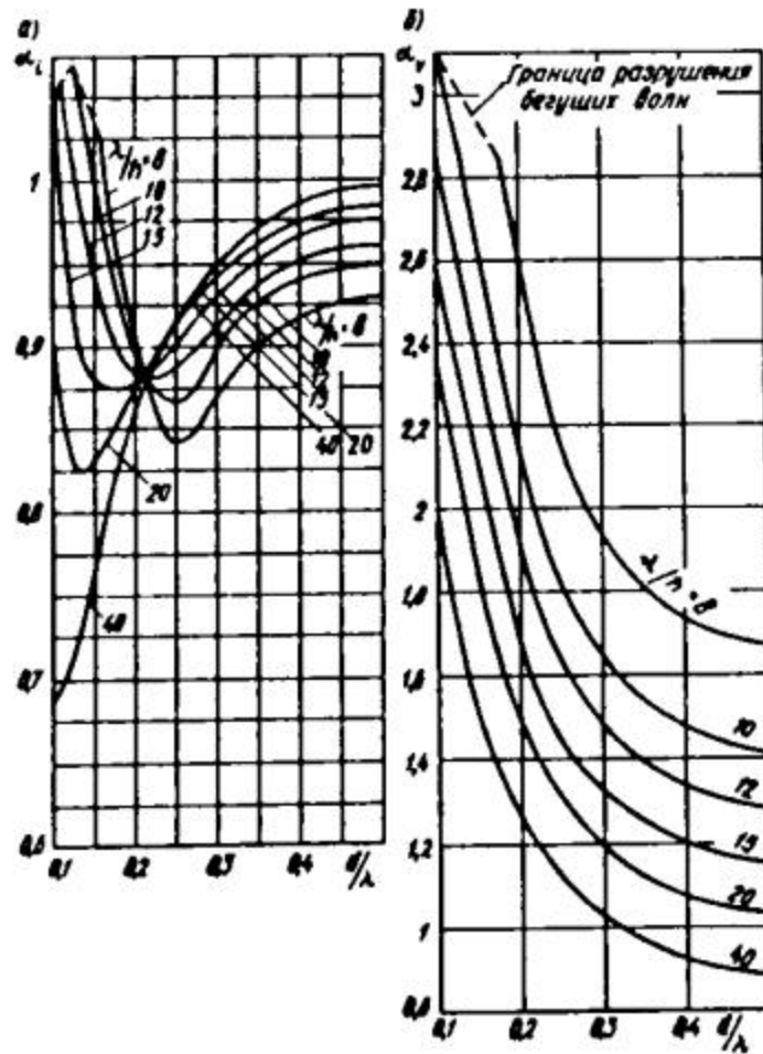
Рис. 16. Графики значений инерционного a_i и скоростного a_v коэффициентов глубины
