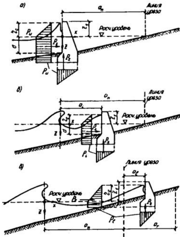
Рис. 27. Эпюры волнового давления на вертикальную волнозащитную стену при расположении сооружения:
