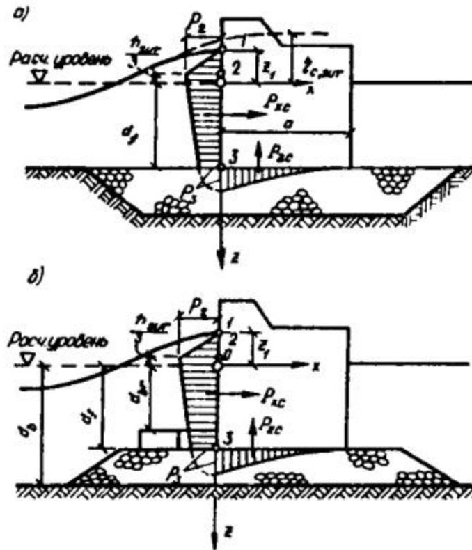
Рис. 9. Эпюры давления прибойных волн на вертикальную стену
