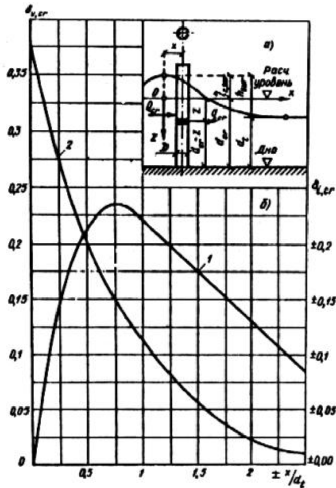
Рис. 24. Схема к определению нагрузок от разбивающихся волн и графики значений коэффициентов d_{i,cr} - кривая 1 и d_{v,cr} - кривая 2
