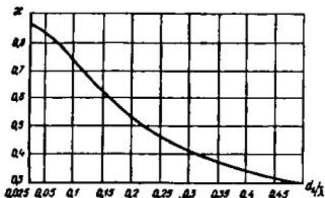
Рис. 32. График значений коэффициента c
