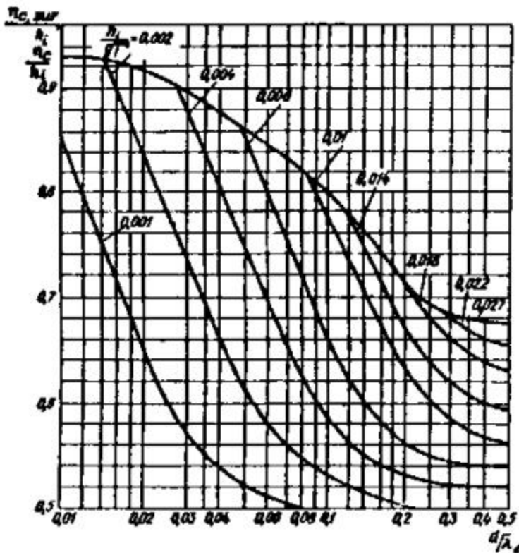
Рис. 3. Графики для определения значений h_c/h_i в мелководной и h_{c,s}V_r/h_i в прибойной зонах
